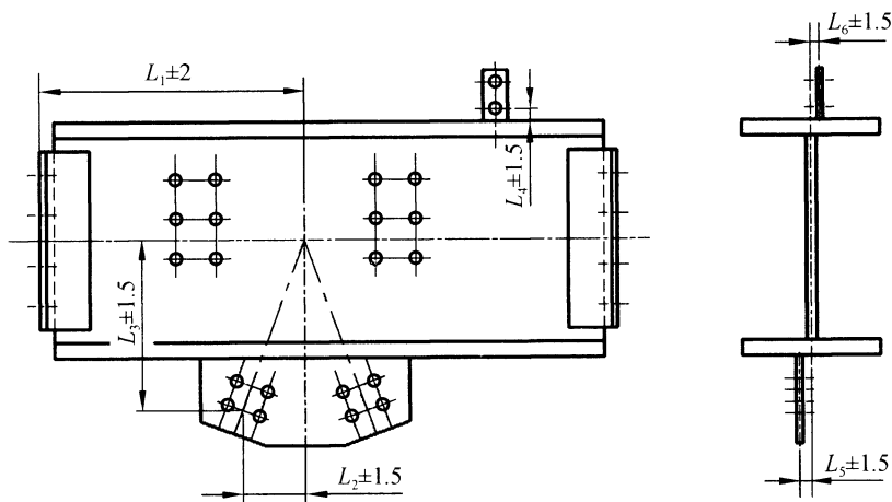
图 11 梁的尺寸偏差（类型 II）
