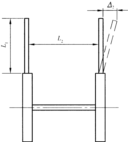
图 17 柱上连接板的尺寸偏差
