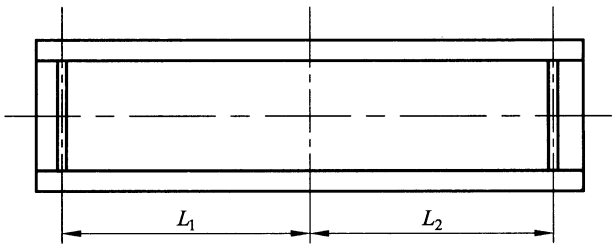
图 5 顶板主梁支承间的长度偏差
