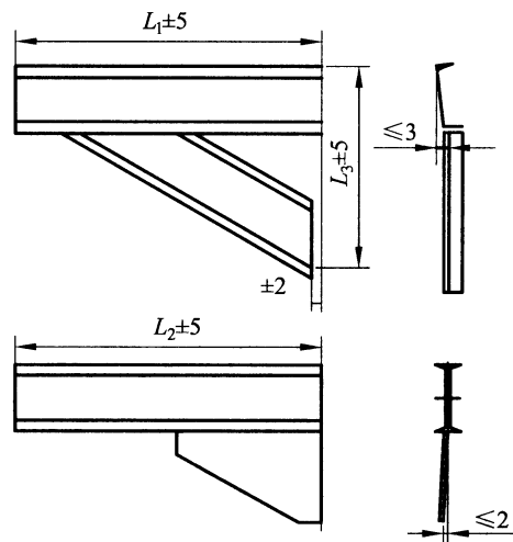
图 24 撑架的尺寸偏差
