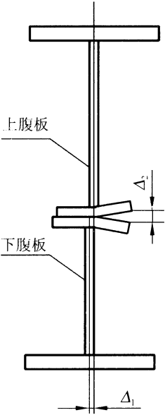
图 18 叠梁的偏差
