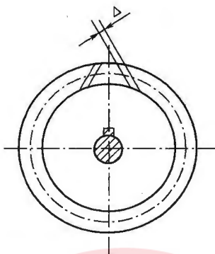
图 7.1.1-2 链轮的齿尖错位 Δ—同一轴上任意两链轮齿尖前后错位
