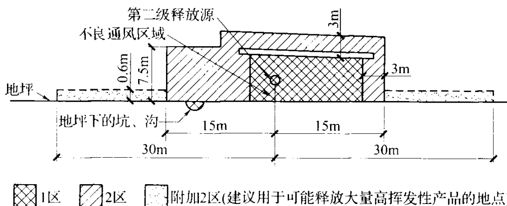
图 B. 0. 1-3 可燃物质重于空气、释放源在封闭建筑物内通风不良的生产装置区
