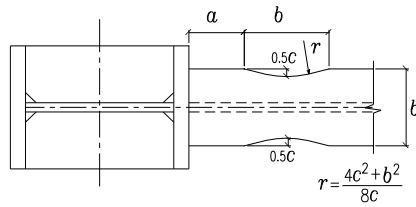
图 17.3.8 骨形节点
