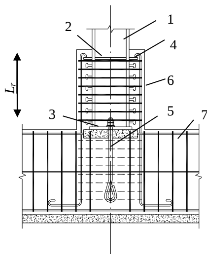
图 12.7.7 外包式柱脚
