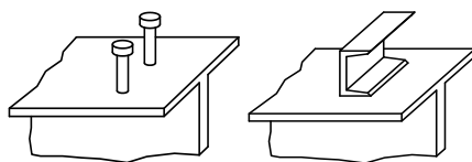
(a) 圆柱头焊钉连接件 (b) 槽钢连接件
